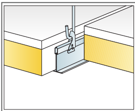
Techo colgado con varilla y Clip de cuelgue
